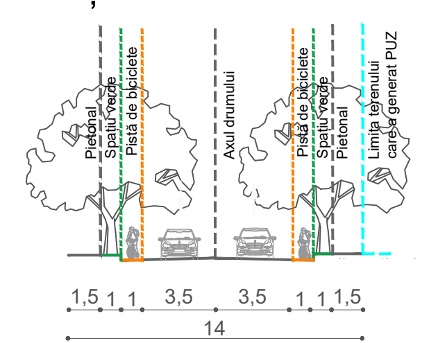
SECȚIUNE B-B' PROPUȘĂ
