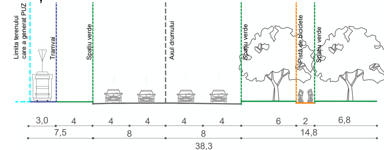
SECȚIUNE CEALEA ZIMANDULUI A-A' sc. 1:250 - existent
