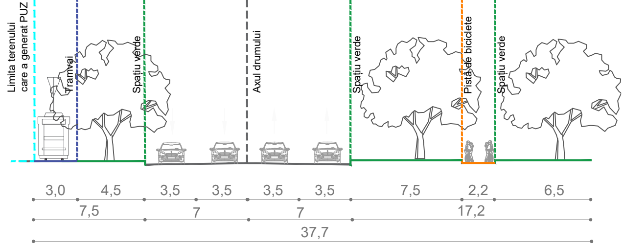
SECȚIUNE CALEA ZIMANDULUI A-A' sc. 1:250- existent
